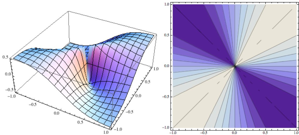
図 2: f(x,y) = \frac{xy}{x^2 + y^2} のグラフと等高線
