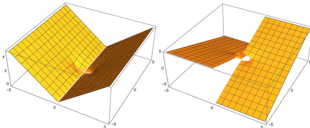
図 13: \text{p.v.}\sqrt{z^2-1} の実部・虚部のグラフ (左半平面で \varphi(z) と異なる)
