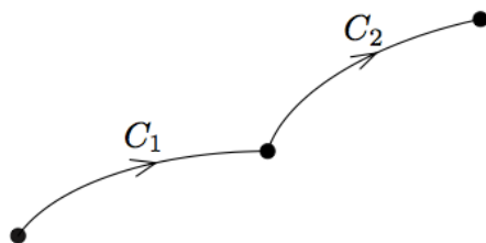
図 16: C_1 の終点 = C_2 の始点ならば C_1 + C_2 が作れる
