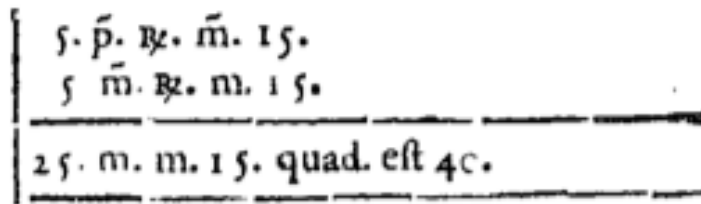
図 1: 足して 10, かけて 40 となる 2 数は 5 \pm \sqrt{-15} (Ars Magna から)
