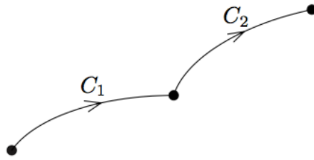
図 6: C_1 の終点 = C_2 の始点ならば C_1 + C_2 が作れる
