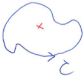
図 24: \int_C f(z) dz \neq 0 かも
