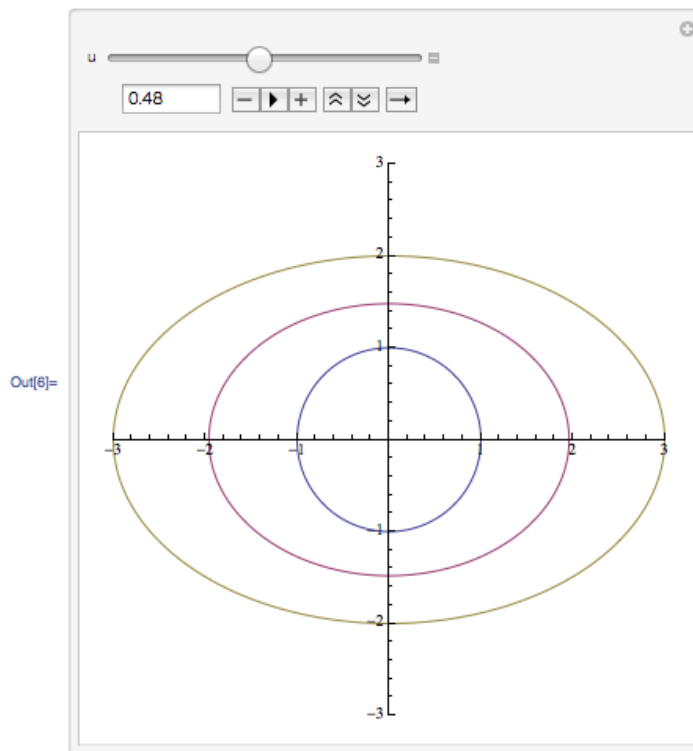
図 30: 円 \varphi_0(t) = (\cos t, \sin t) を楕円 \varphi_1(t) = (3 \cos t, 2 \sin t) に連続的に変形
