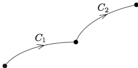
図 7: C_1 の終点 = C_2 の始点ならば C_1 + C_2 が作れる
