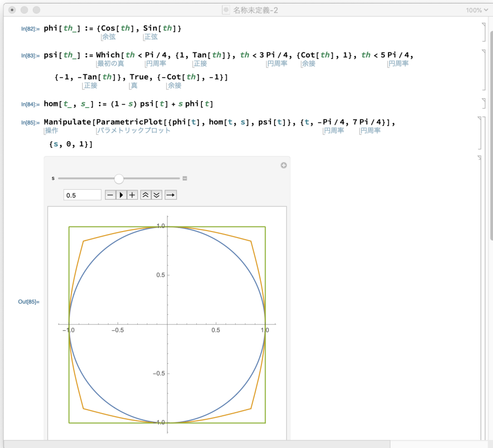
図 20: 正方形の周 \Gamma を円周 C に連続的に変形する
