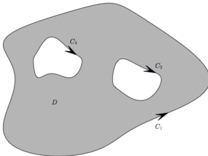
図 19: 領域 D の境界 \partial D は C_1 + C_2 + C_3 に等しい
