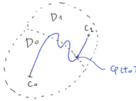
図 21: c_0 から c_1 に至る道、最後に D_0 を出るところ \varphi(t_0)
