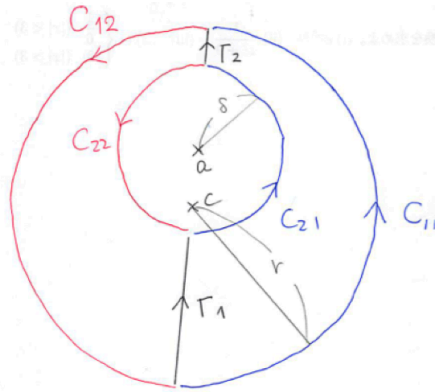
図 11: 切り込みを入れて二つの閉曲線の和として表す
