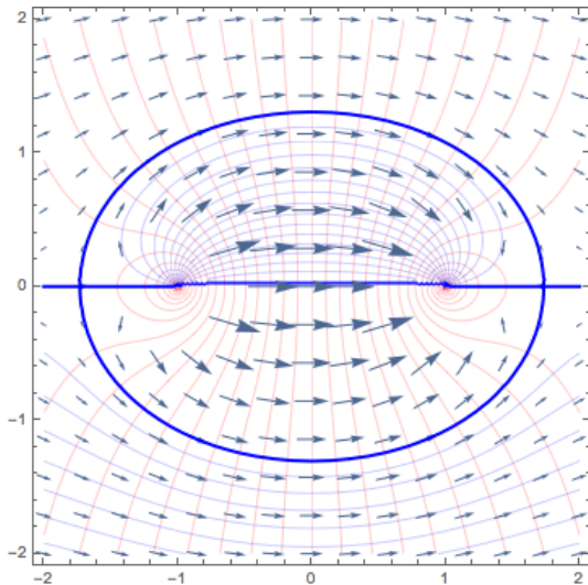
Figure: Rankine の卵形 (同じ強さの湧き出し・吸い込みと一様流の重ね合わせ)
