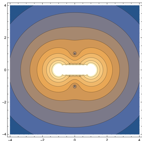
図 12: 21 点複合シンプソン公式の誤差の特性関数 (絶対値の常用対数)
