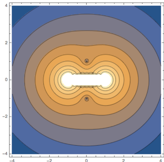
図 5: 21 点複合シンブソン公式の誤差の特性関数 (絶対値の常用対数)
