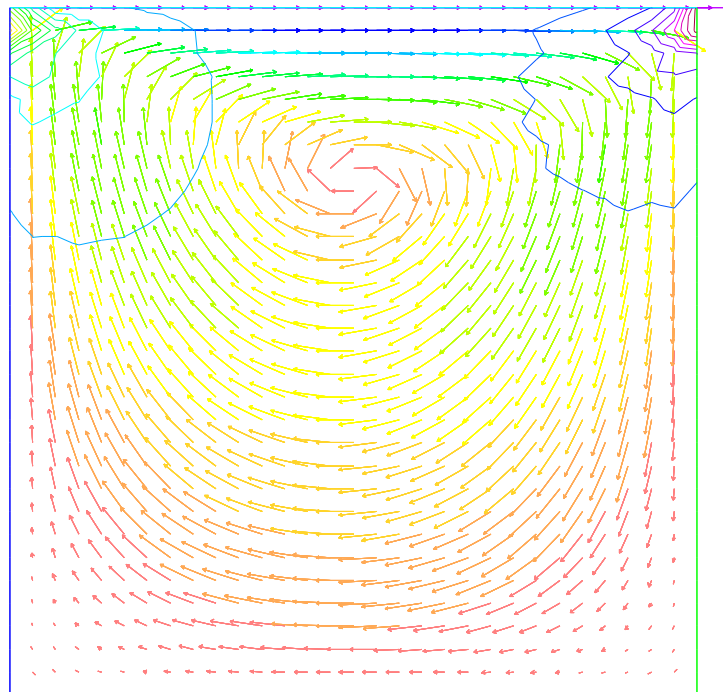
図 6: stokes-p1b.edp の結果
