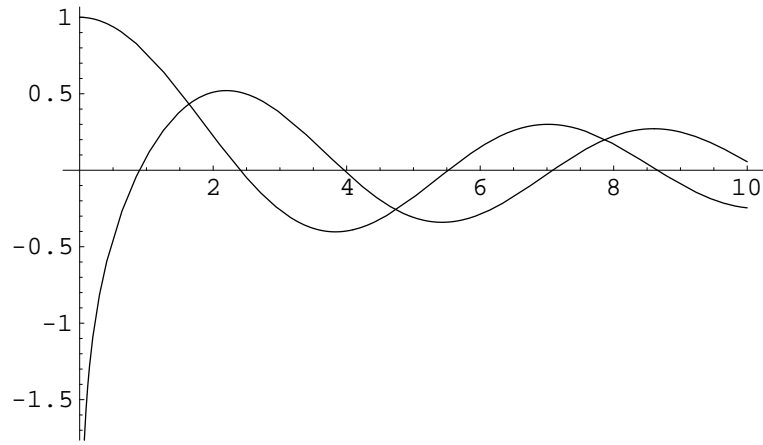
図 2.1: J_0 と Y_0 のグラフ (Plot[{BesselJ[0,x],BesselY[0,x]},{x,0,10}])
