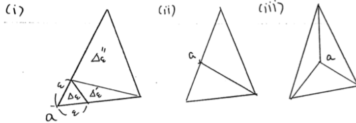
図 17: a が三角形 \Delta のどこにあるかで場合分け (頂点, 边上, 内部)
