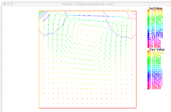
図 1: Stokes-cavity.edp の実行結果
